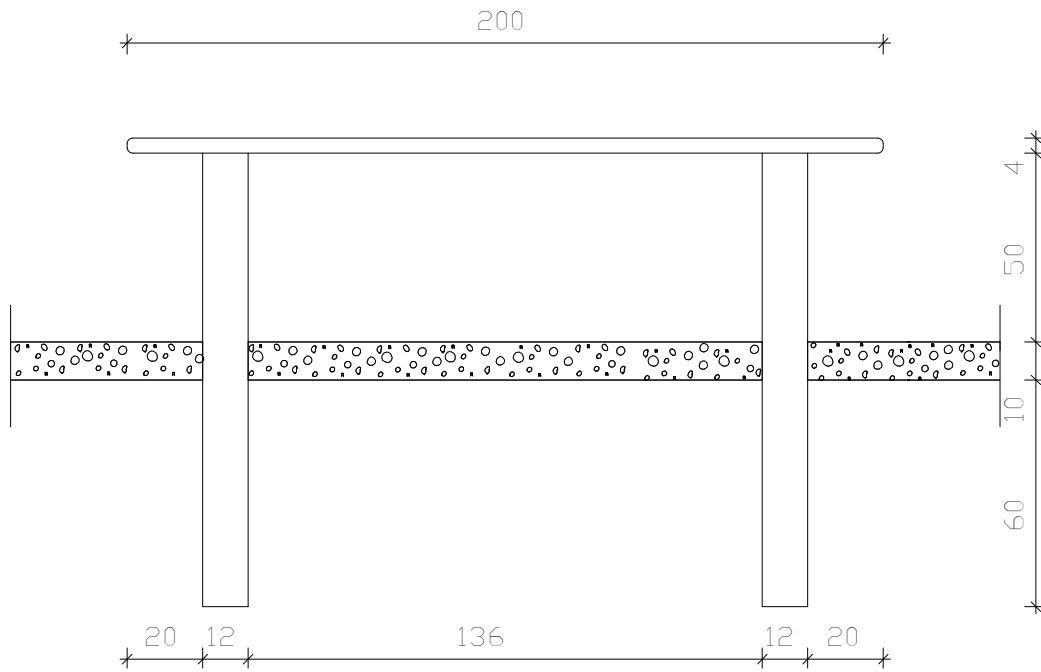
WIDOK FRONTOWY
